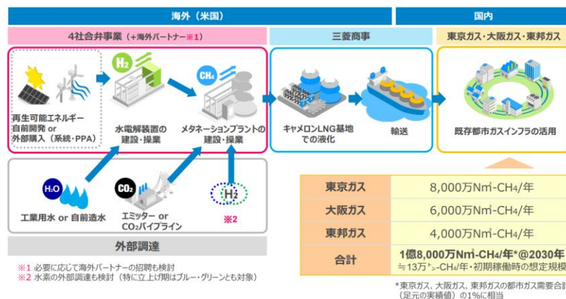
《図表 2-10》 日本への合成メタン導入スキーム (検討例)
